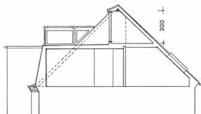
TVÆRSNIT A-A
